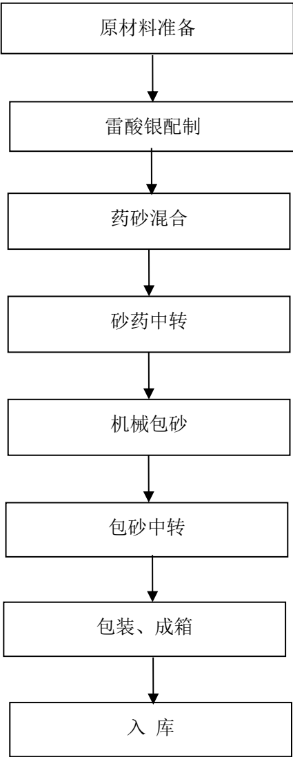
图 2. 4-5 玩具类（摩擦型/砂炮）产品生产工艺流程图
