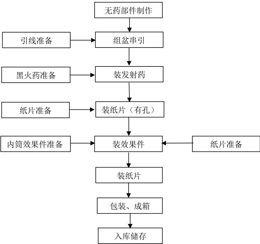
图 2.4-3 组合烟花类产品生产工艺流程图
