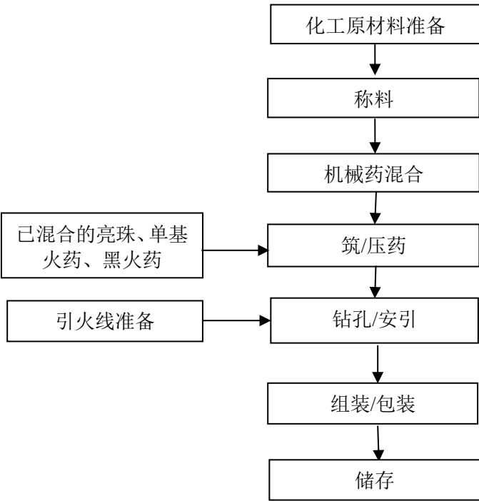
图 2.4-4 喷花类产品生产工艺流程图
